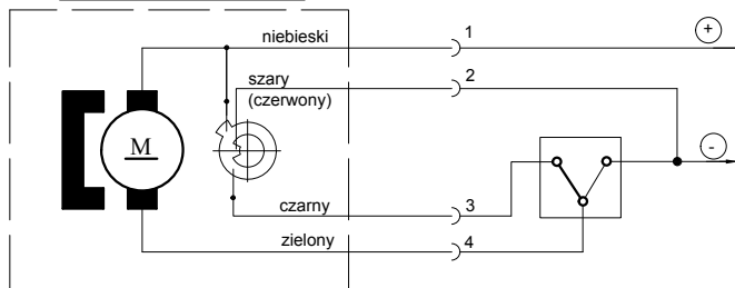
Schemat elektryczny
