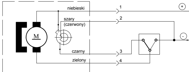
Schemat elektryczny
